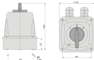
max. liczba segmentów-4 z dławicami PG16
